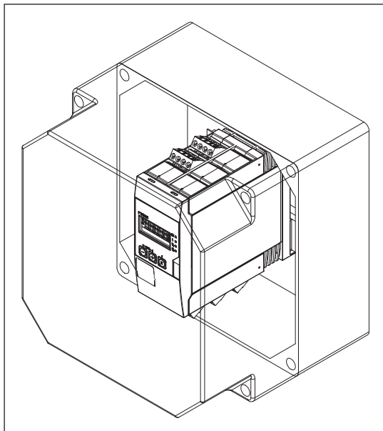
10 Schutzgehäuse für Hutschienengeräte
