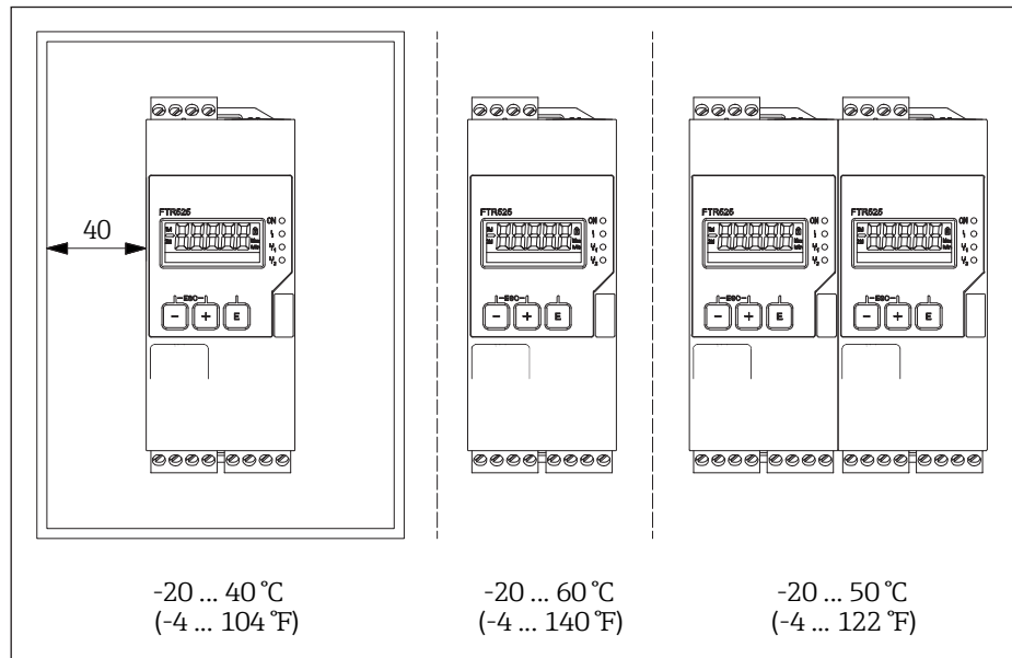
4 Zulässige Umgebungstemperaturen am FTR525
