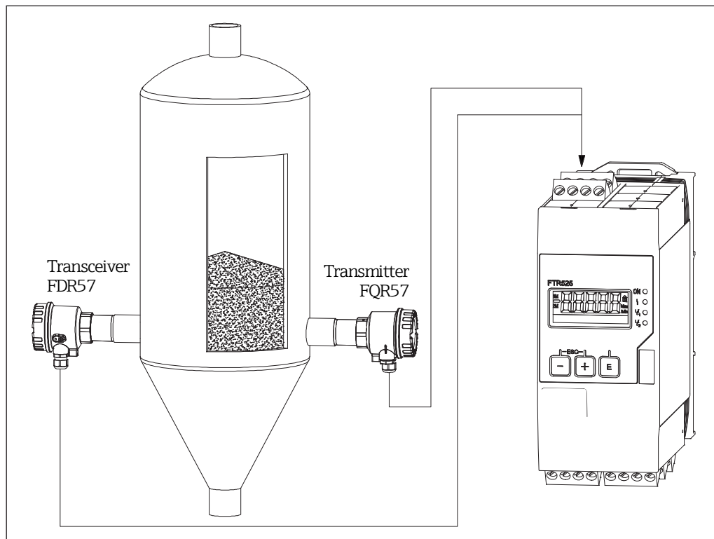
1 Beispiel Grenzstanddetektion
