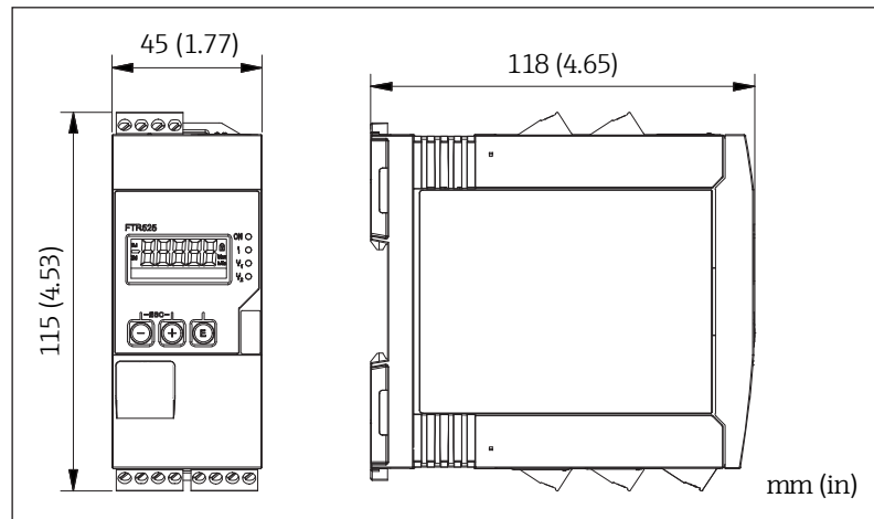
5 Abmessungen des FTR525
