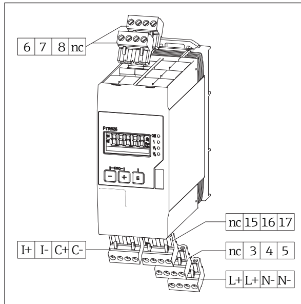
2 Klemmenbelegung des FTR525
