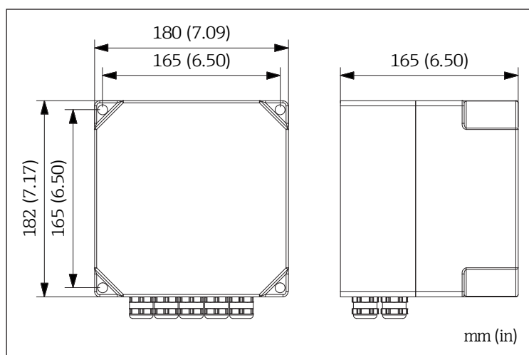
11 Abmessungen Schutzgehäuse
