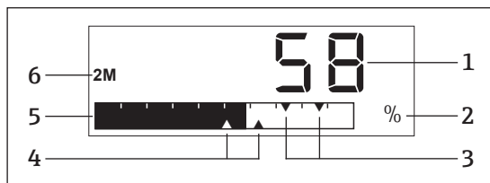
☑ 7 Beispiel Messwertanzeige bei Geräteausführung mit zwei Relaisausgängen
